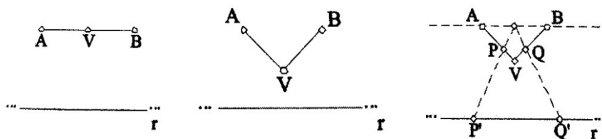
Figura 5: Correspondencia biunívoca entre segmento y recta (Fuente: Arrigo, D'Amore y Sbaragli, 2011, p. 101)
