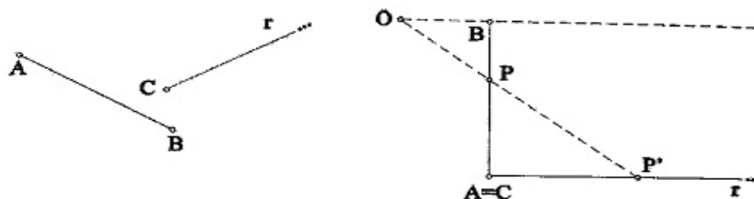
Figura 4: Correspondencia biunívoca entre segmento y semirrecta (Fuente: Arrigo, D'Amore y Sbaragli, 2011, p. 101)
