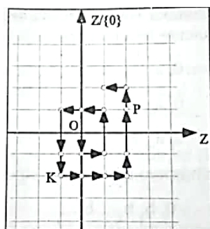
Figura 7: Correspondencia biunívoca entre \mathbb{N} y \mathbb{Q} (Fuente: Arrigo, D'Amore y Sbaragli, 2011, p. 111)
