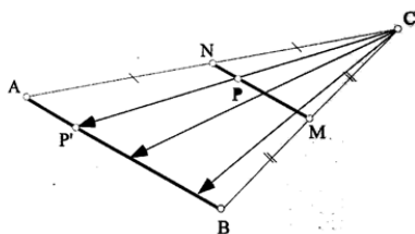
Figura 1: Correspondencia biunívoca entre dos segmentos (Fuente: Arrigo, D’Amore y Sbaragli, 2011, p. 55)
